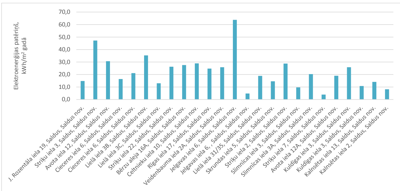
2.30. att. Īpatnējais elektroenerģijas patēriņš Saldus pilsētas pašvaldības ēkās, 2019
