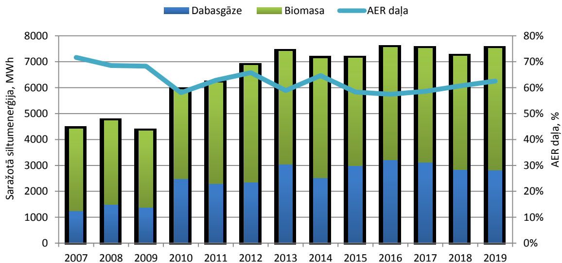
2.16. att. Kurināmā sadalījums Saldus novada vietējos siltumenerģijas ražošanas avotos
