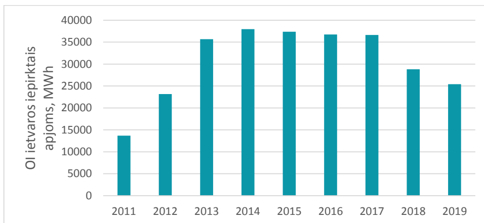
2.20. att. Saražotā elektroenerģija Saldus novadā (OI iepirktais apjoms)
