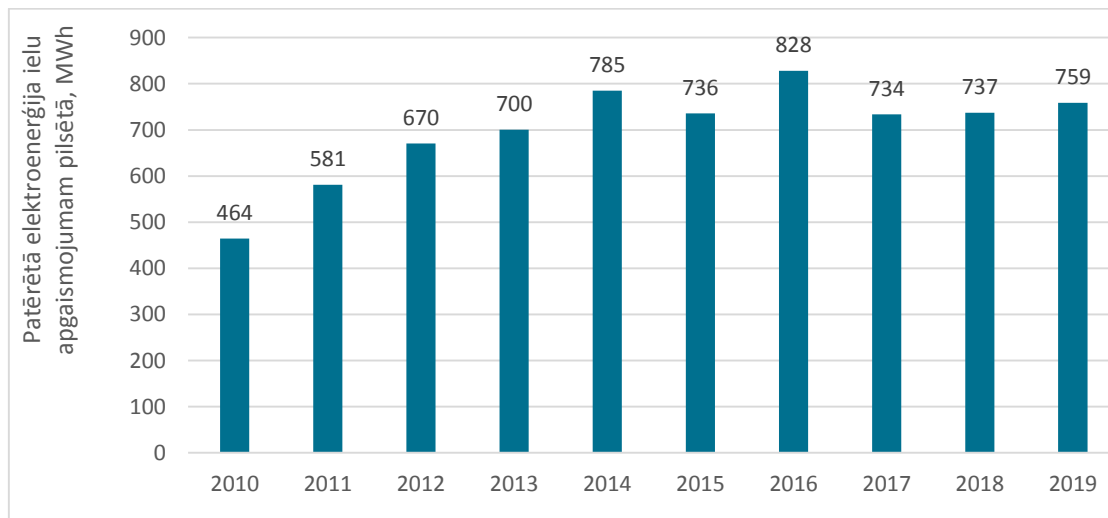
2.32. att. Elektroenerģijas patēriņš ielu apgaismojumam Saldus pilsētā
