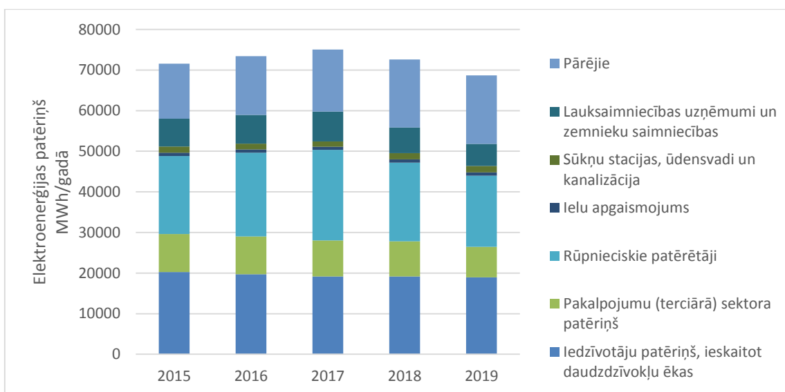
2.29. att. Elektroenerģijas patēriņa sadalījums galapatērētājos 10
