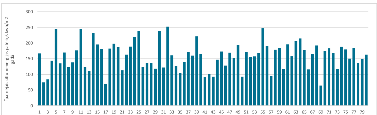
2.26. att. Īpatnējais siltumenerģijas patēriņš daudzdzīvokļu ēkās Saldus pilsētā, par kurām ir pieejami dati par 2019. gadu
