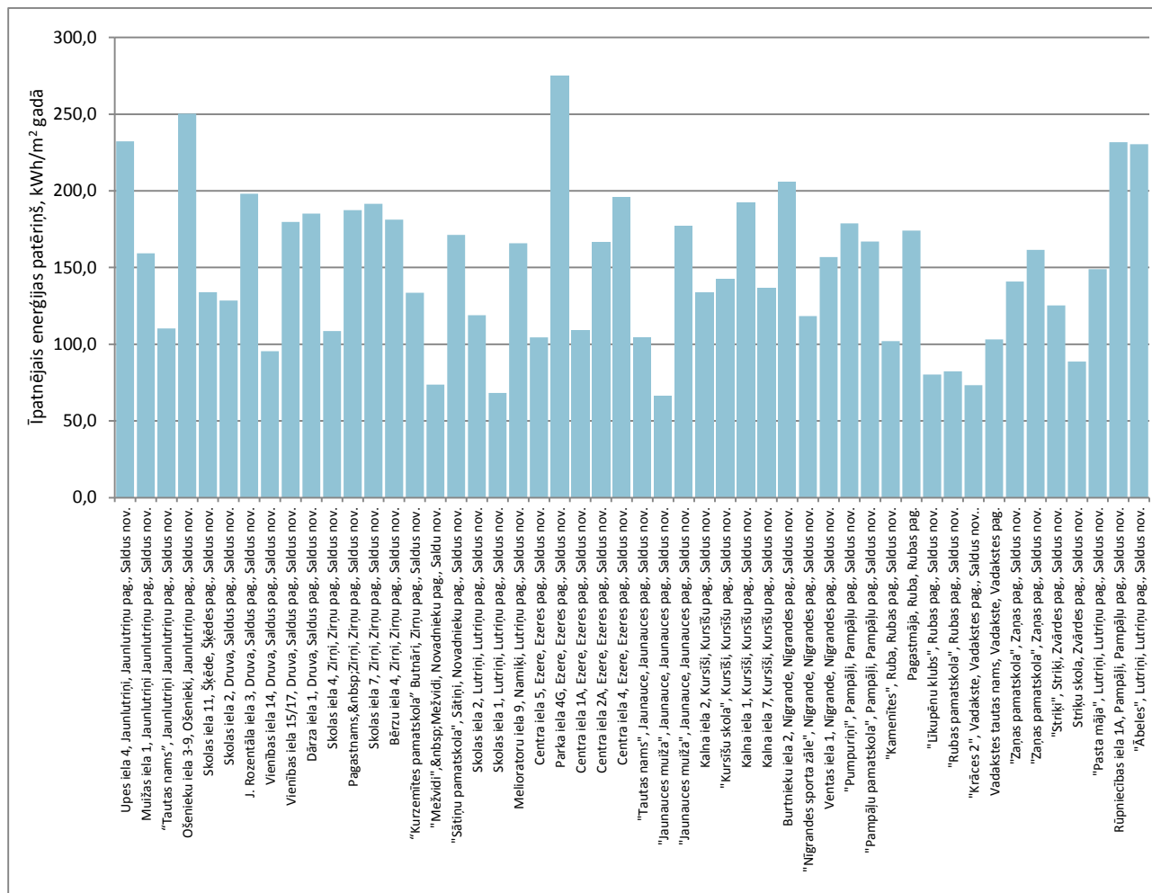
2.24. att. Īpatnējais enerģijas patēriņš Saldus novada pašvaldības pagastu ēkās 2019. gadā
