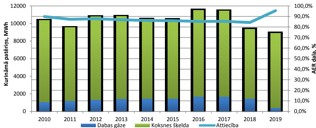
2.14. att. Kurināmā veida un patēriņa sadalījums Saldus novada ciemu CSS
