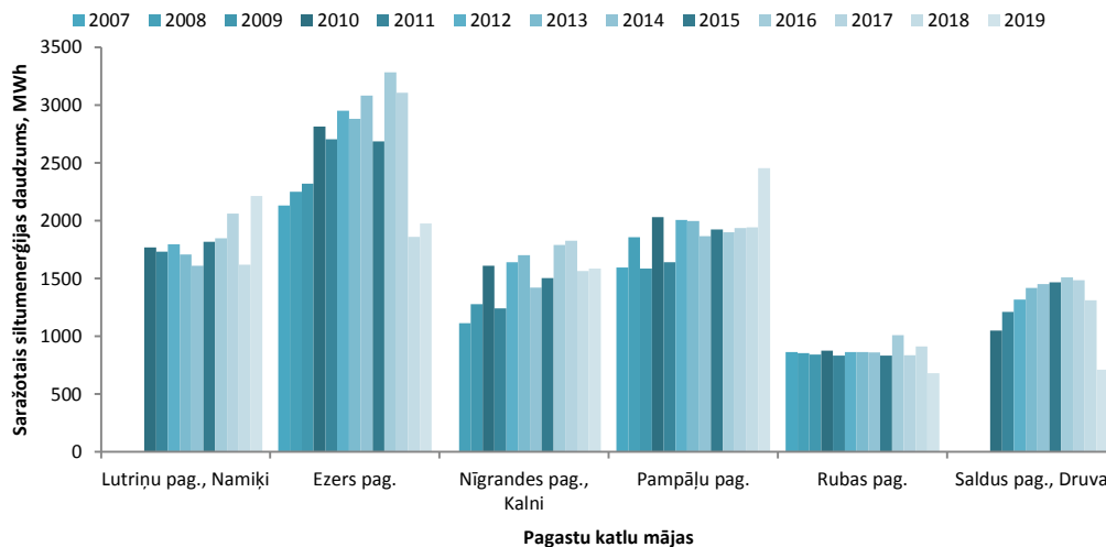
2.13. att. Saldus novada ciemu katlu māju raksturojums
